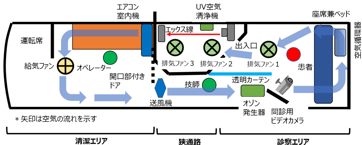
図2 上から見た車内の空気の流れ
