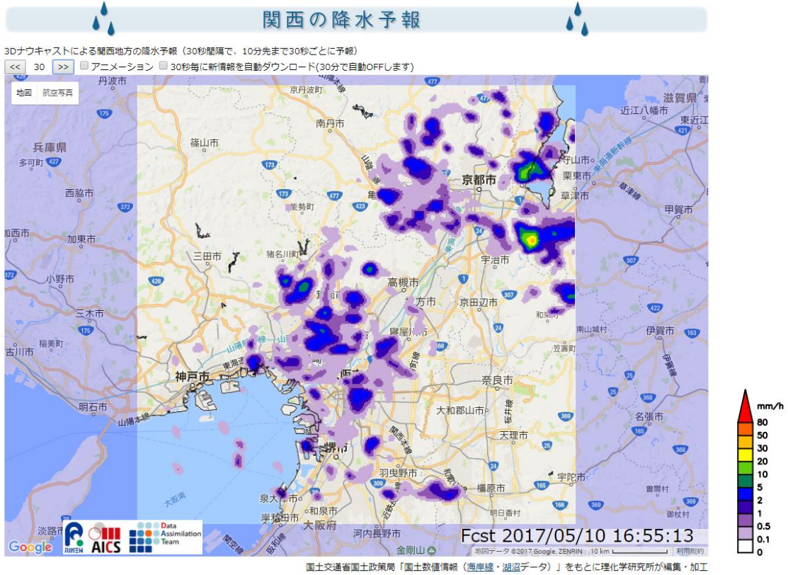
図1 10分後の降水分布予報の例
